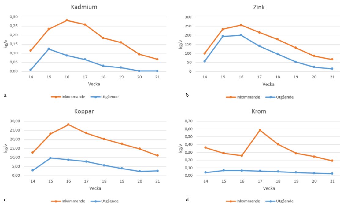
Figur 9. Massflöden i kg/vecka av inkommande och utgående metallmängder vid reningsverket. Här ses liknande trender för zink, koppar och kadmium, när inkommande avloppsvattenflöde är högt inkommer stora mängder av dessa metaller till reningsverken.
