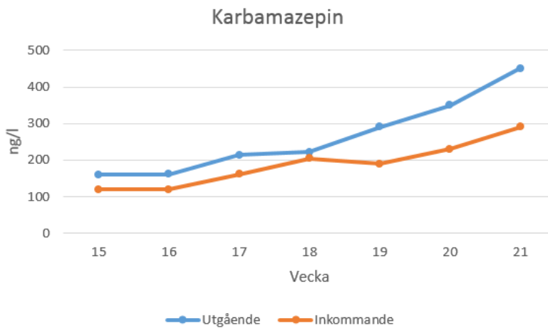
Figur 5. Inkommande och utgående halter av Karbamazepin, ett antiepileptika, på Främby under provtagningsperioden.
