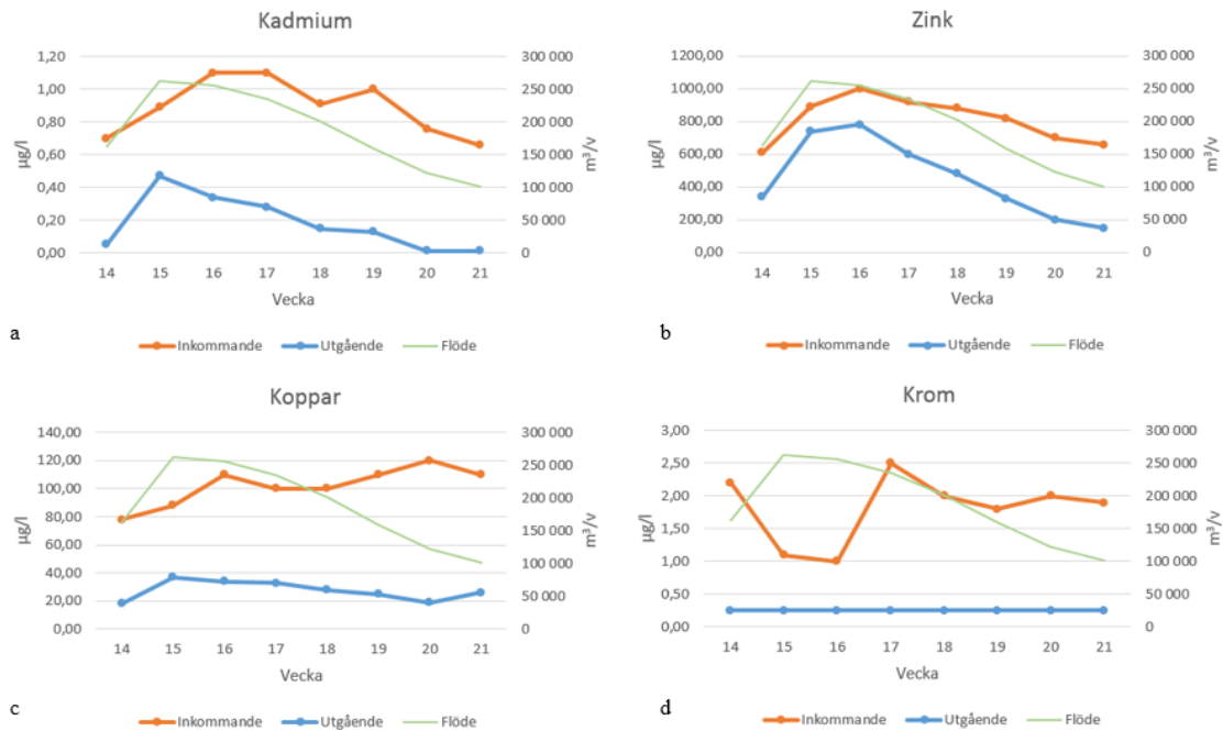
Figur 4. Inkommande och utgående halter från veckoprovtagningen av zink, kadmium, krom och koppar på Främby reningsverk under provtagningsperioden.
